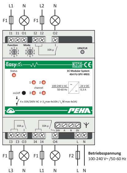
Ausgang 1-4 ⇔ Kanal 1-4 ⇔ LED 1-4
